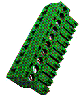
Abbildung 3: Schraubklemmenstecker für CN7. Steckertyp: Phoenix PTR AKZ 1550 Rm 3.81 10 Pol. / Artikel-Nr. F4405
